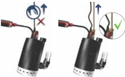
Fig. 5 Izado de la bomba
