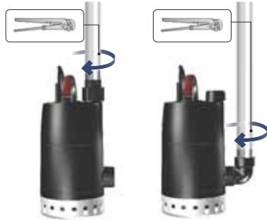
Fig. 7 Conexión de la tubería de descarga
