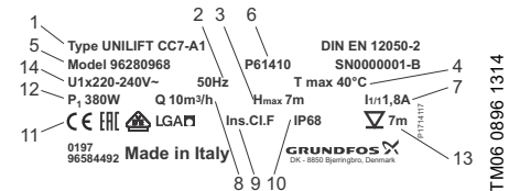
Fig. 16 Ejemplo de placa de características
